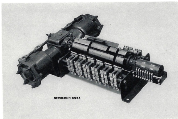
Inverseur de marche. — Wendeschalter. — Reversing switch. Inversor de marcha.
