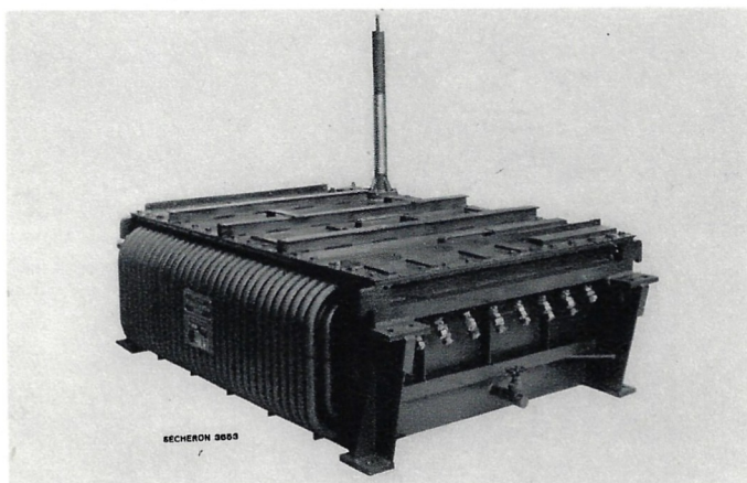
Transformateur à gradins. — Stufentransformator. — Tapped Transformer. Transformador escalonado.
