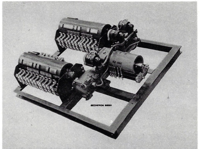
Inverseur de marche. Wendeswitcher. Reversing-switch.
