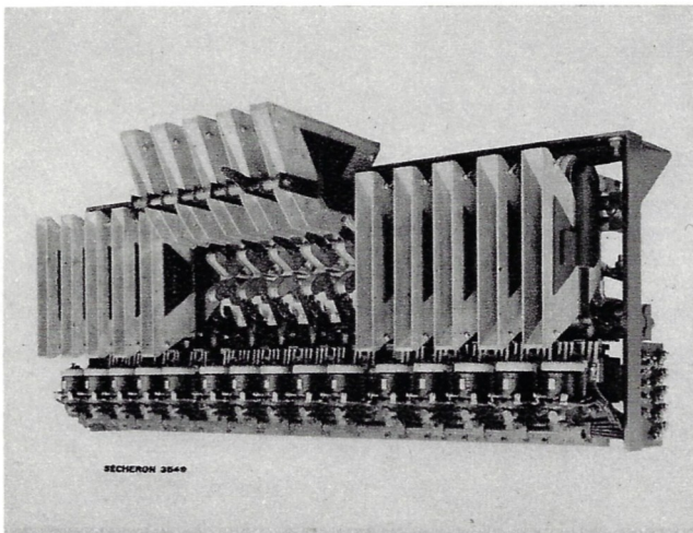
Batterie de contacteurs. Hüpferbatterie. Contactor unit.
